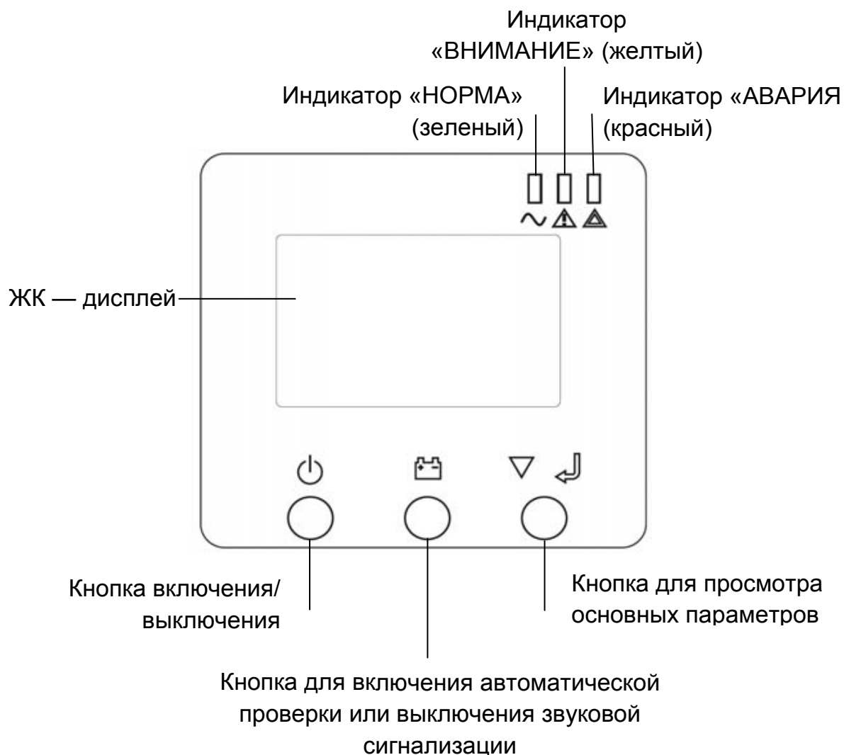
Рисунок 1 – передняя панель изделия
