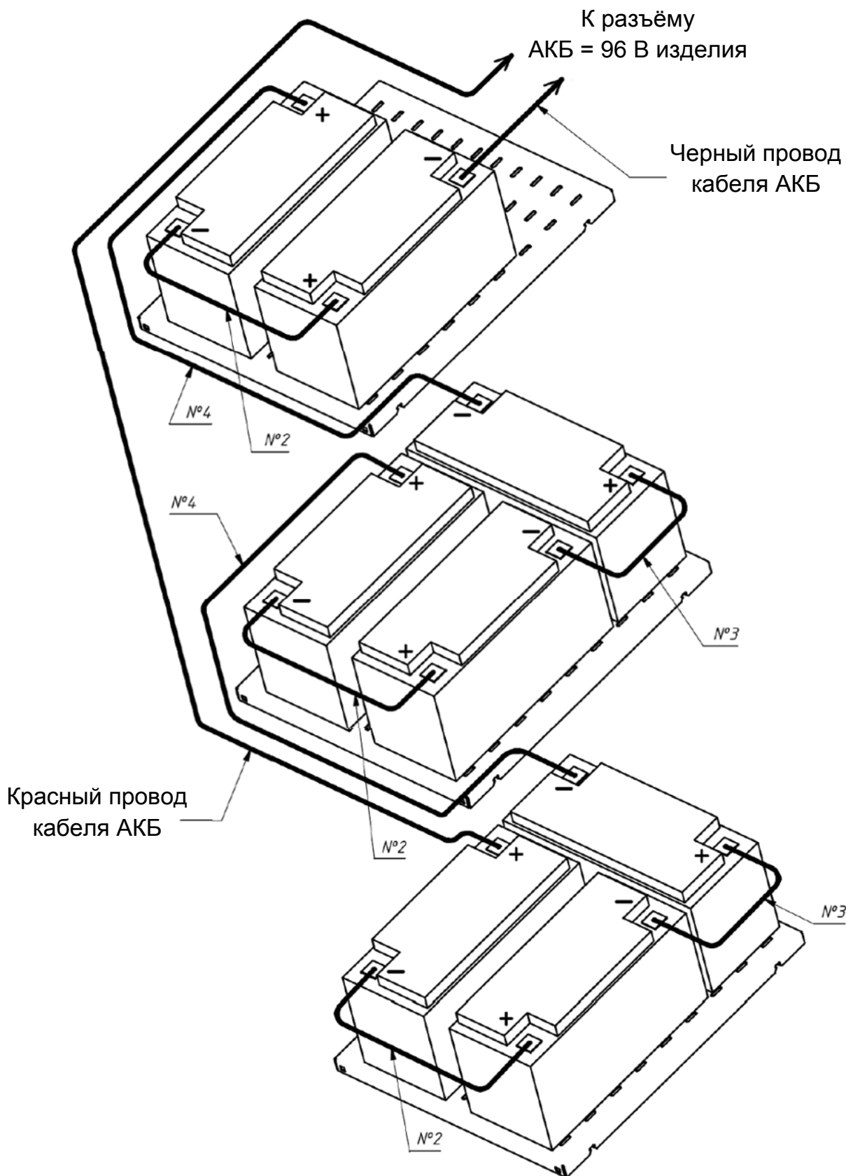
Рисунок 5. Размещение АКБ на полках шкафа и соединение их перемычками.
