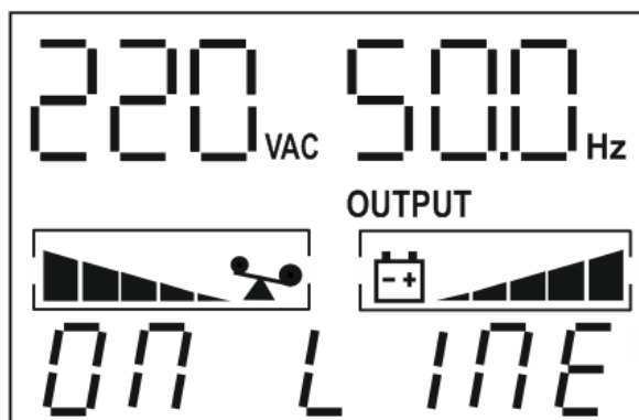
Рисунок 2 – основной экран ЖК-дисплея в режиме «ОСНОВНОЙ»
