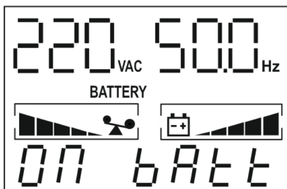
Рисунок 3 – основной экран ЖК-дисплея в режиме «РЕЗЕРВ»
