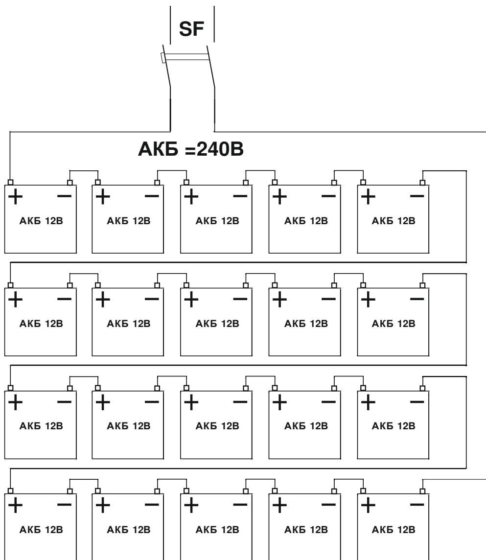
Рисунок 5 – схема монтажа аккумуляторной батареи
