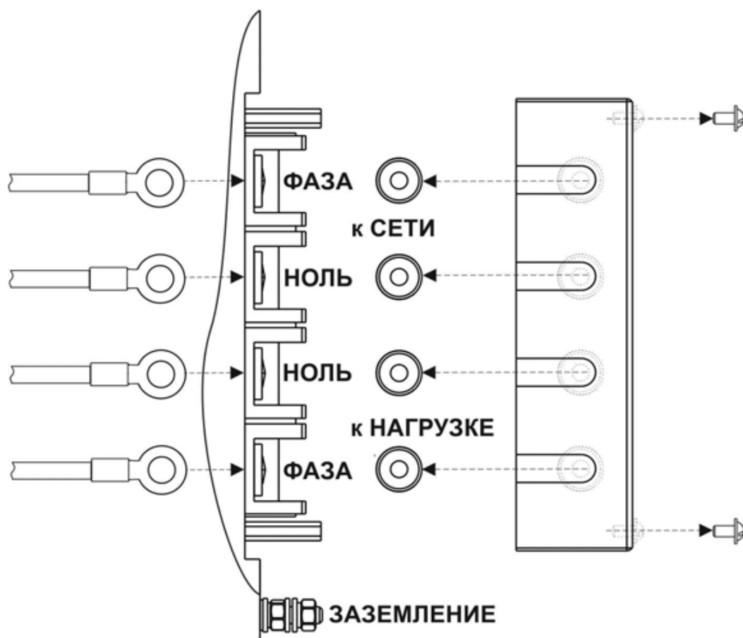
Рисунок 3 – Подключение изделия
