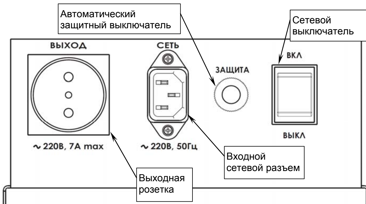
Рисунок 3 – Вид стабилизатора со стороны подключения
