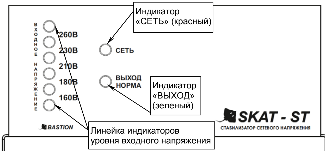
Рисунок 2 – Вид стабилизатора со стороны индикации
